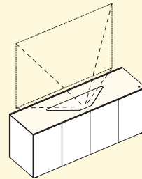
MEDIA-BACKBOARD MIT PROJEKTOR MEDIA CREDENZA WITH INTEGRATED PROJECTOR B/L: 120 / 160 / 200 / 240 H: 82 T/P: 60
